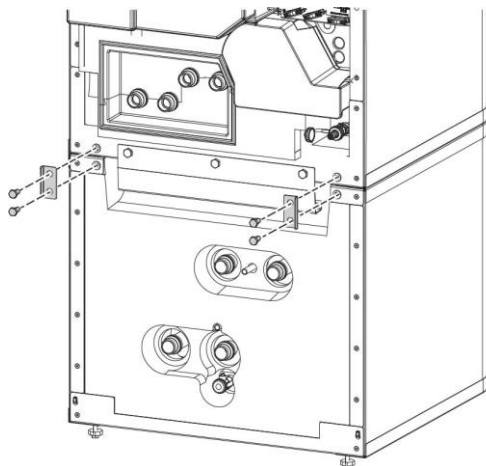
Abbildung 39: Lösen der Verbindungsschrauben
