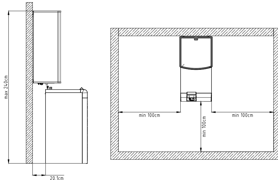
Abbildung 67: Montageanweisung AIR BASIC mit ECO-Speicher
