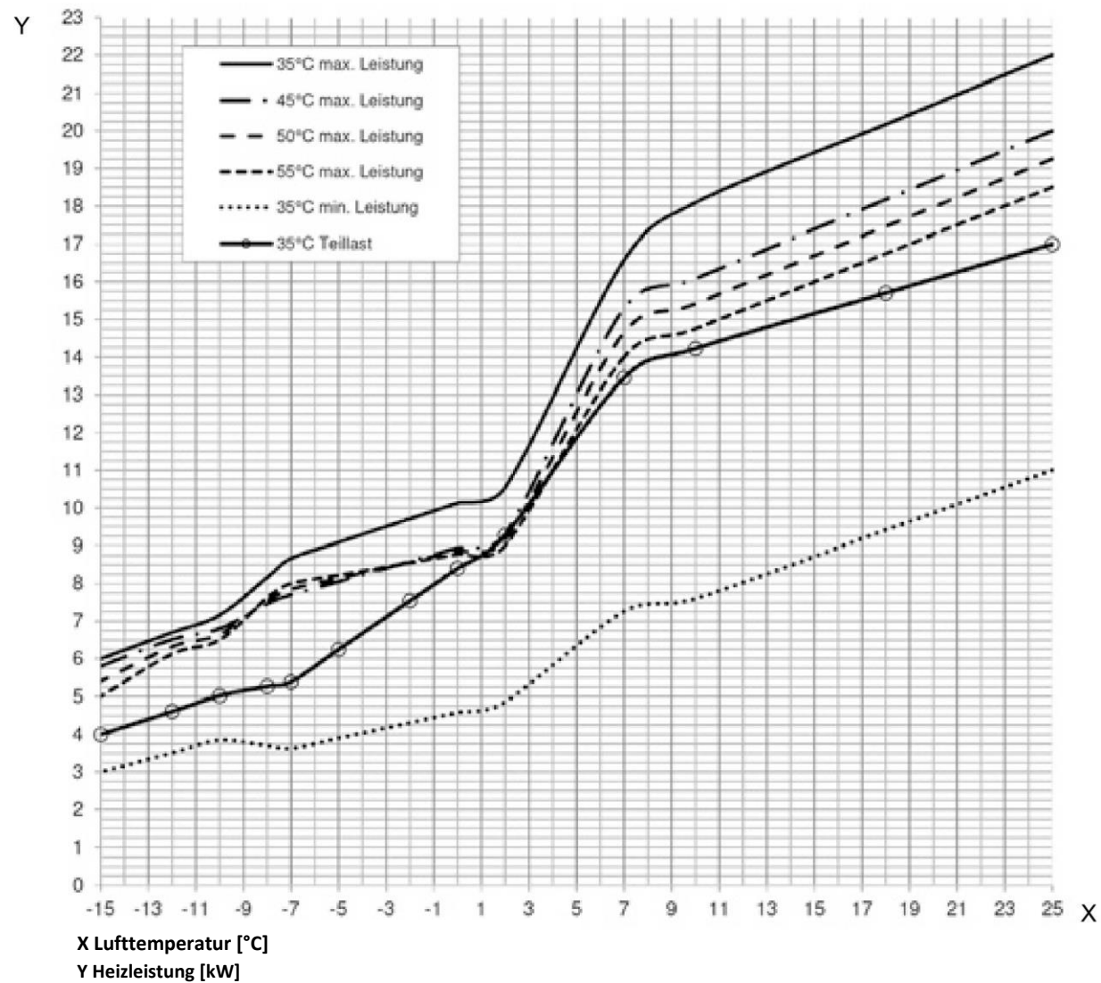
Abbildung 72: Leistungskurve AIR BASIC 618
