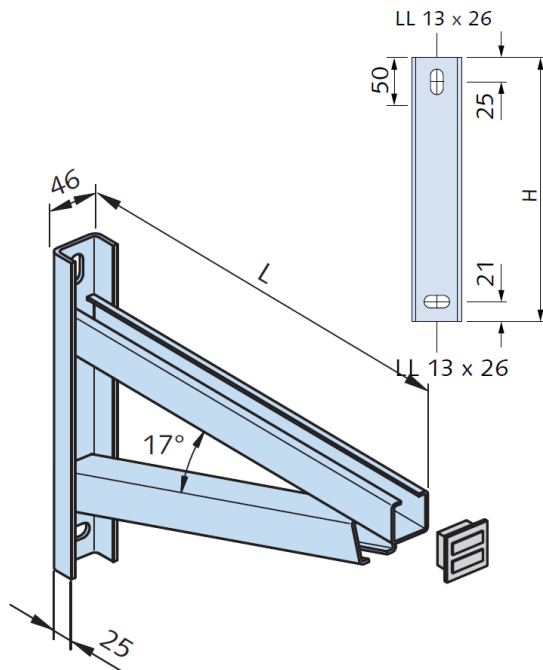
Abbildung 11: Abmessungen Wandkonsole
