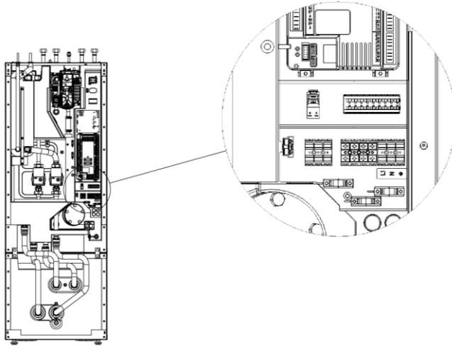
Abbildung 48: Anschluss Elektrik T200
