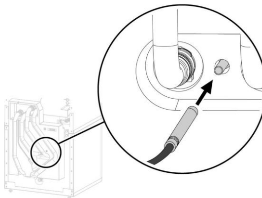
Abbildung 36: Fühler aus Pufferspeicher ziehen
