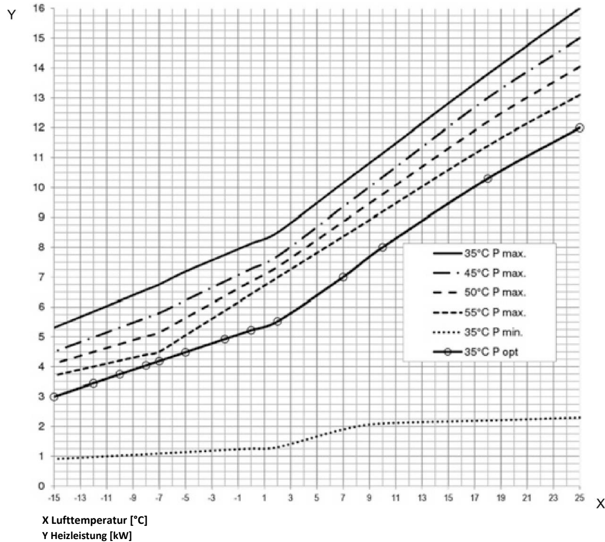
Abbildung 70: Leistungskurve AIR BASIC 211
