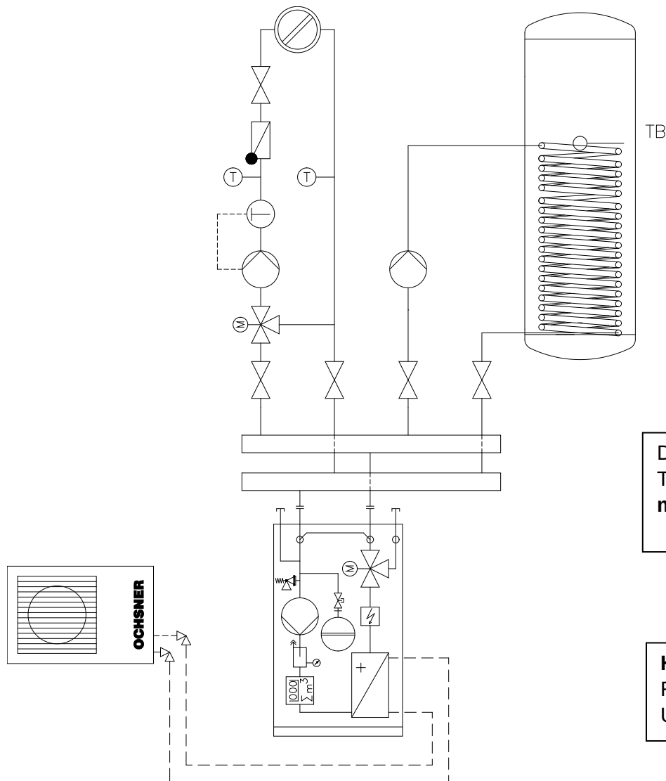
Abbildung 29: Anlagenschema Hydraulik Variante IV
