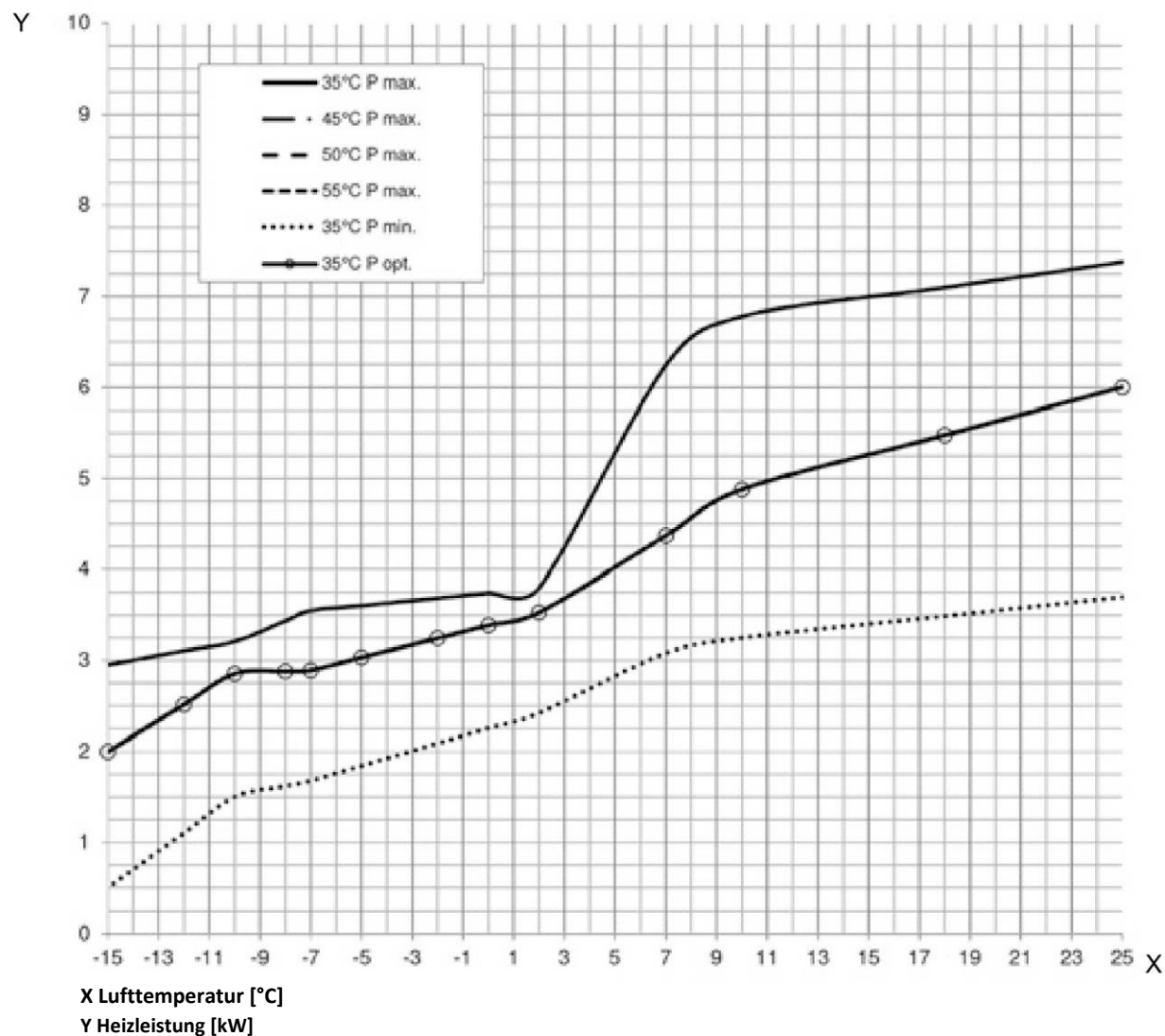
Abbildung 69: Leistungskurve AIR BASIC 109
