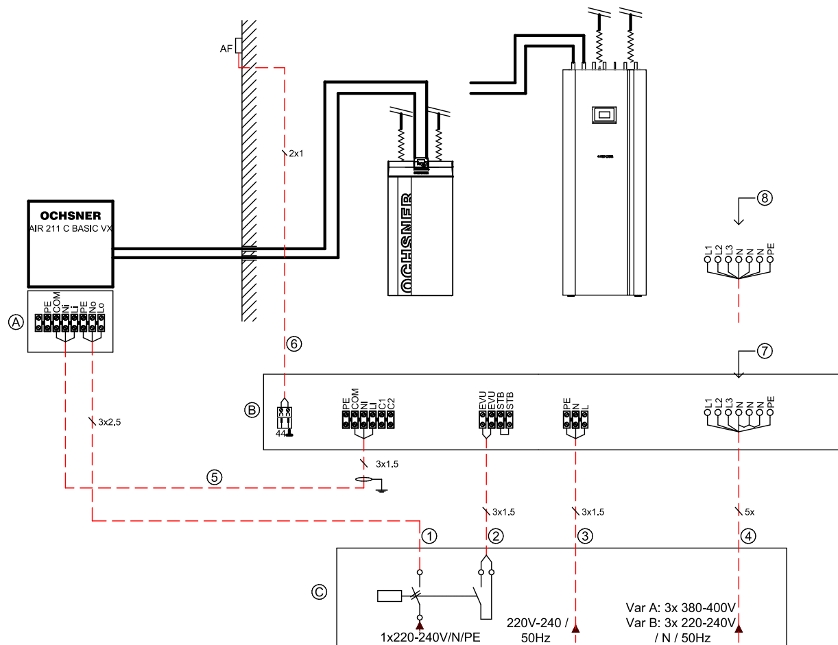
Abbildung 62: Verkabelungsschema AIR BASIC 211 (unterbrechbare Versorgung Innenteil über Außenteil)
