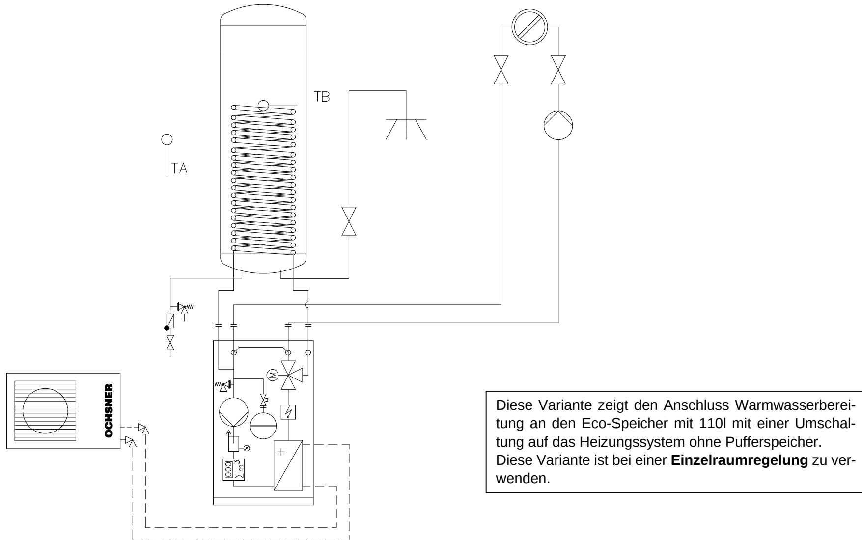
Abbildung 27: Anlagenschema Hydraulik Variante IIa
