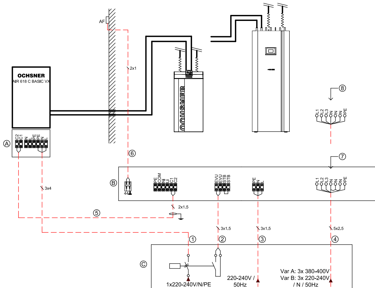
Abbildung 64: Verkabelungsschema AIR BASIC 618
