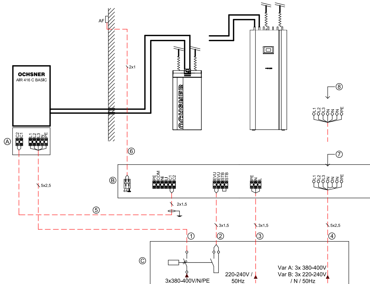
Abbildung 63: Verkabelungsschema AIR BASIC 416
