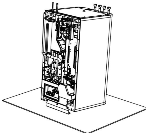
Abbildung 42: Abstellen Oberteil T200
