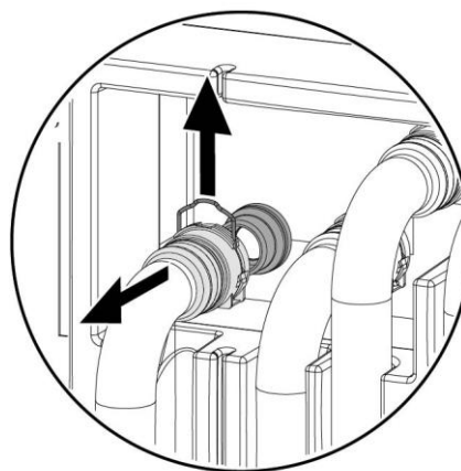
Abbildung 37: Lösen der Steckverbinder
