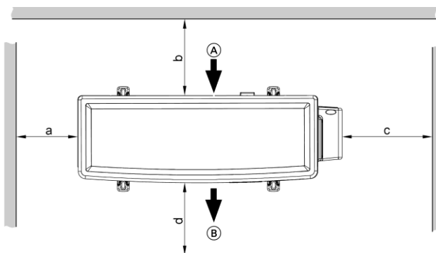
Abbildung 5: Mindestabstände Außenteil
