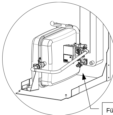
Abbildung 22: Detailansicht Innenteil Füll- und Entleerungshahn
