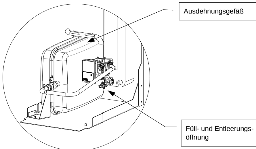
Abbildung 20: Detailansicht Füll- und Entleerung
