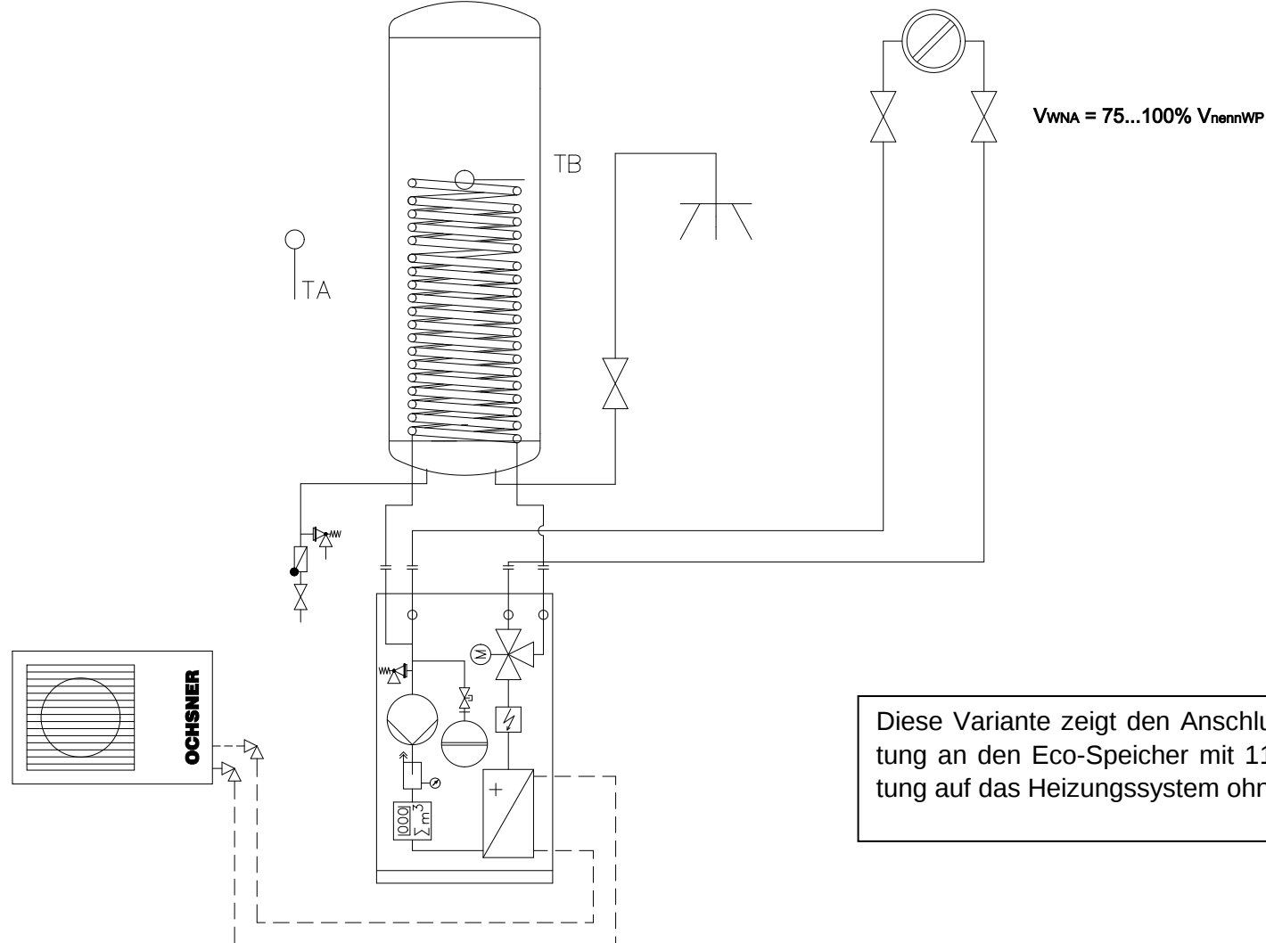
Abbildung 26: Anlagenschema Hydraulik Variante II
