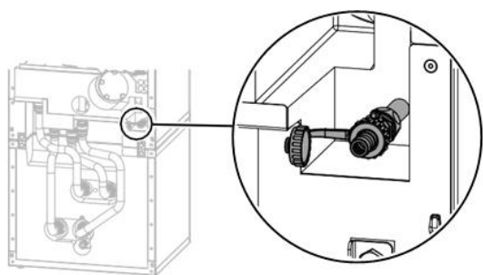
Abbildung 52: Trinkwarmwasser-Speicher entleeren
