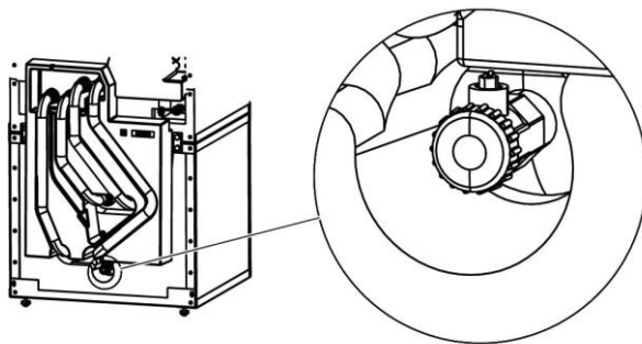
Abbildung 51: Pufferspeicher entleeren
