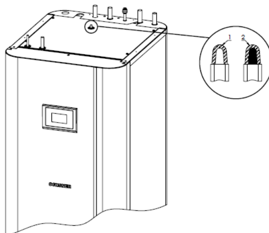
Abbildung 53: Signalanode Trinkwarmwasser-Speicher T200
