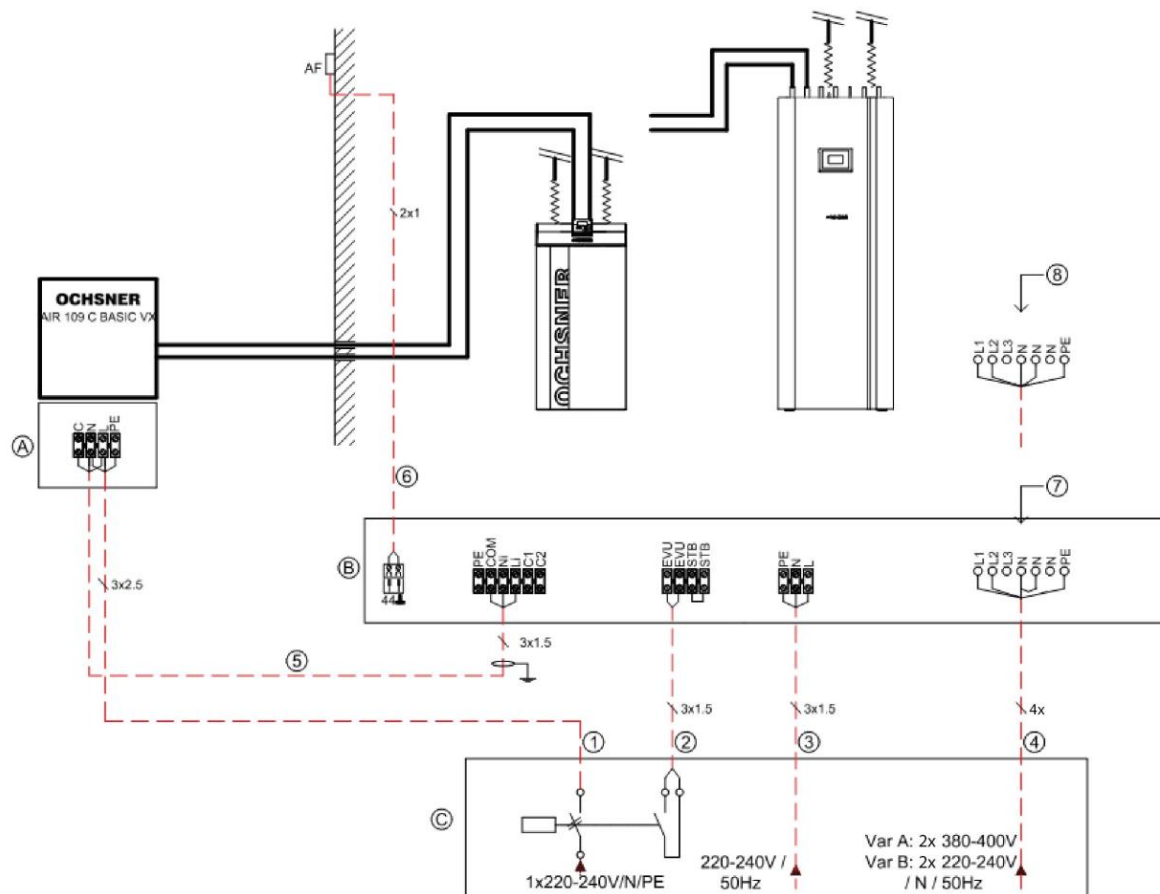
Abbildung 60: Verkabelungsschema AIR BASIC 109 (unterbrechbare Versorgung)
