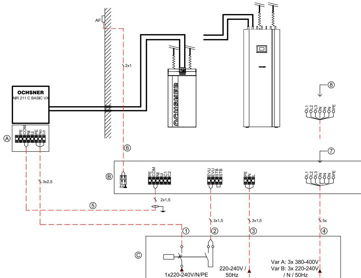
Abbildung 61: Verkabelungsschema AIR BASIC 211
