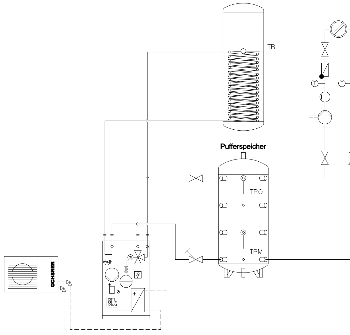
Abbildung 30: Anlagenschema Hydraulik Variante V
