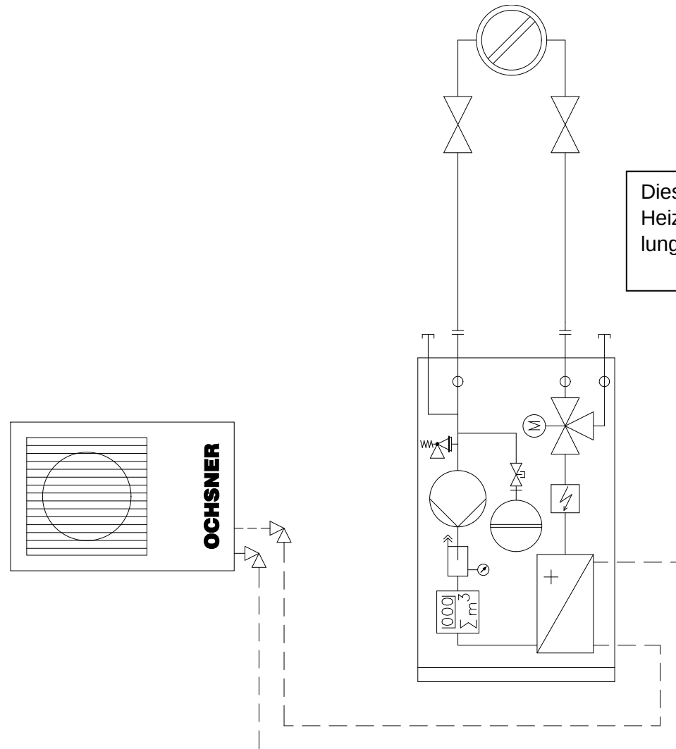
Abbildung 24 Anlagenschema Hydraulik Variante I
