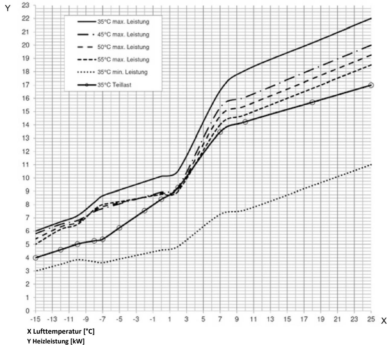
Abbildung 71: Leistungskurve AIR BASIC 416
