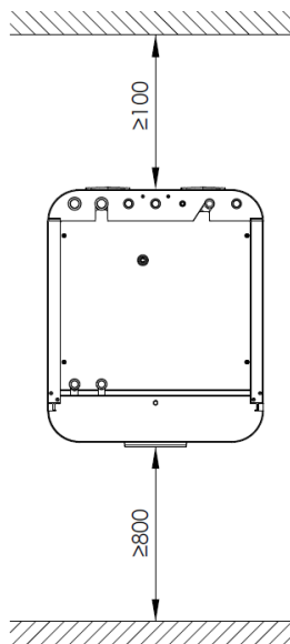
Abbildung 33: Mindestabstände T200
