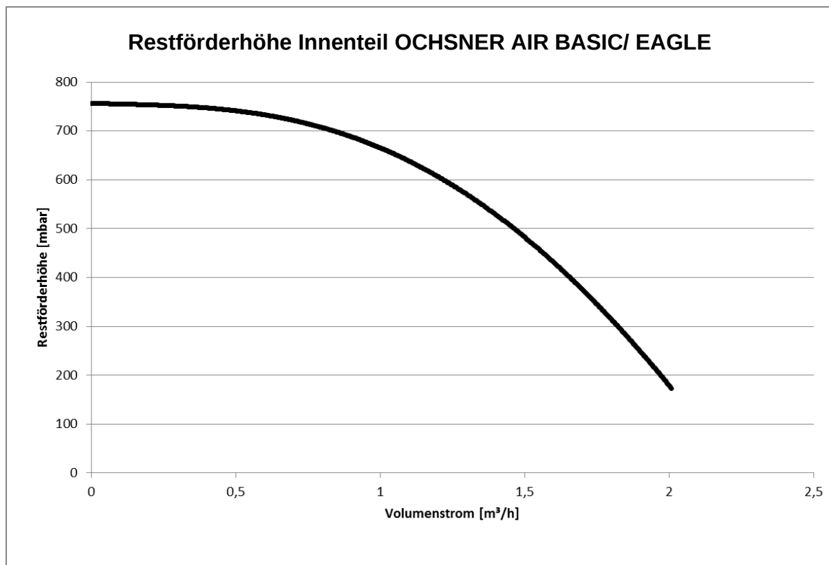
Abbildung 74: Restförderhöhe Innenteil AIR BASIC / EAGLE
