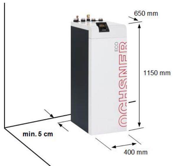
Abbildung 18: Maße Innenteil
