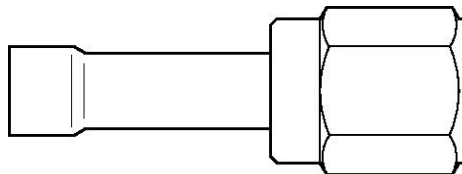
Abbildung 55: Ansicht Löt-Bördelverschraubung
