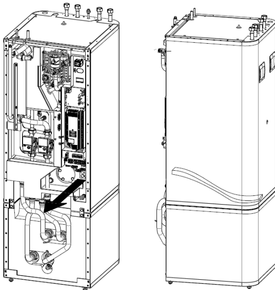
Abbildung 49: Kabeldurchführung Innenteil T200
