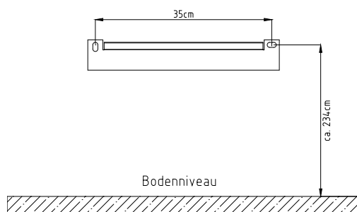
Abbildung 68: Ansicht Befestigungsschiene und Rückansicht Speicher mit Befestigungsschiene
