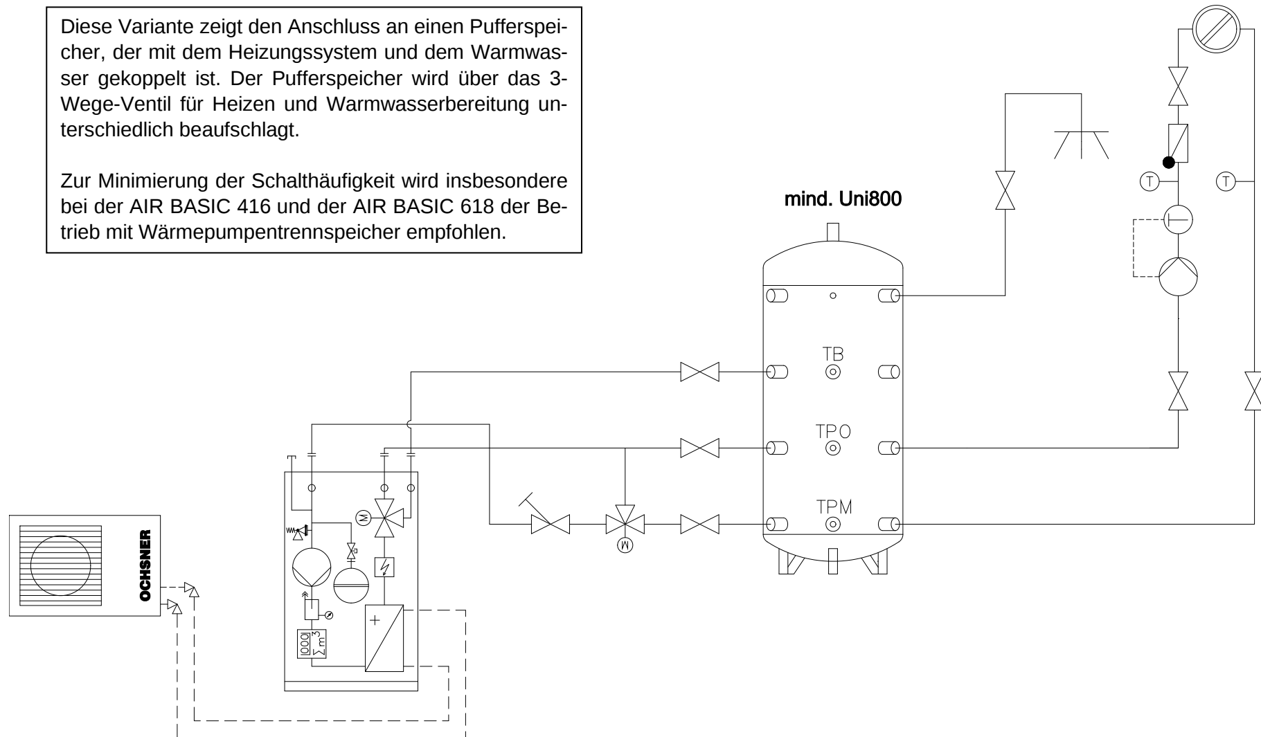
Abbildung 28: Anlagenschema Hydraulik Variante IIIu
