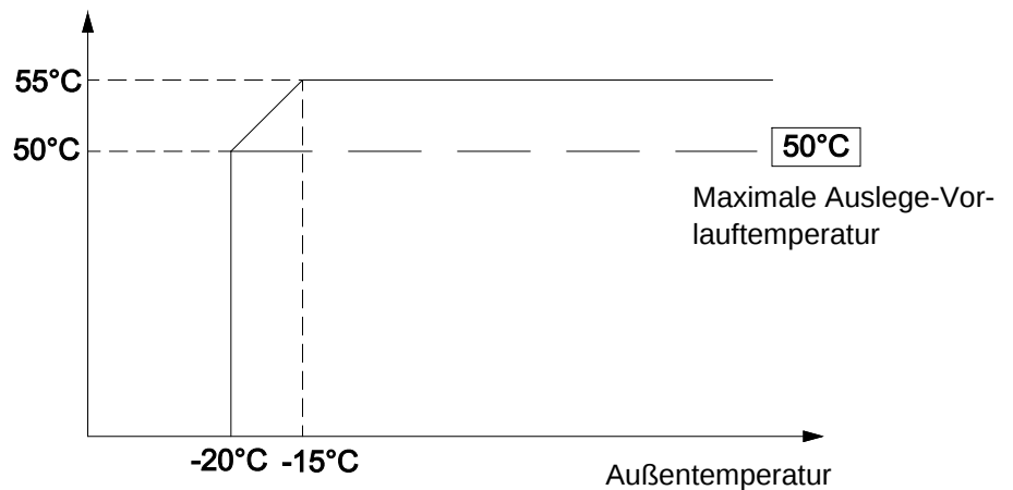
Abbildung 73: Einsatzgrenzen OCHSNER AIR BASIC
