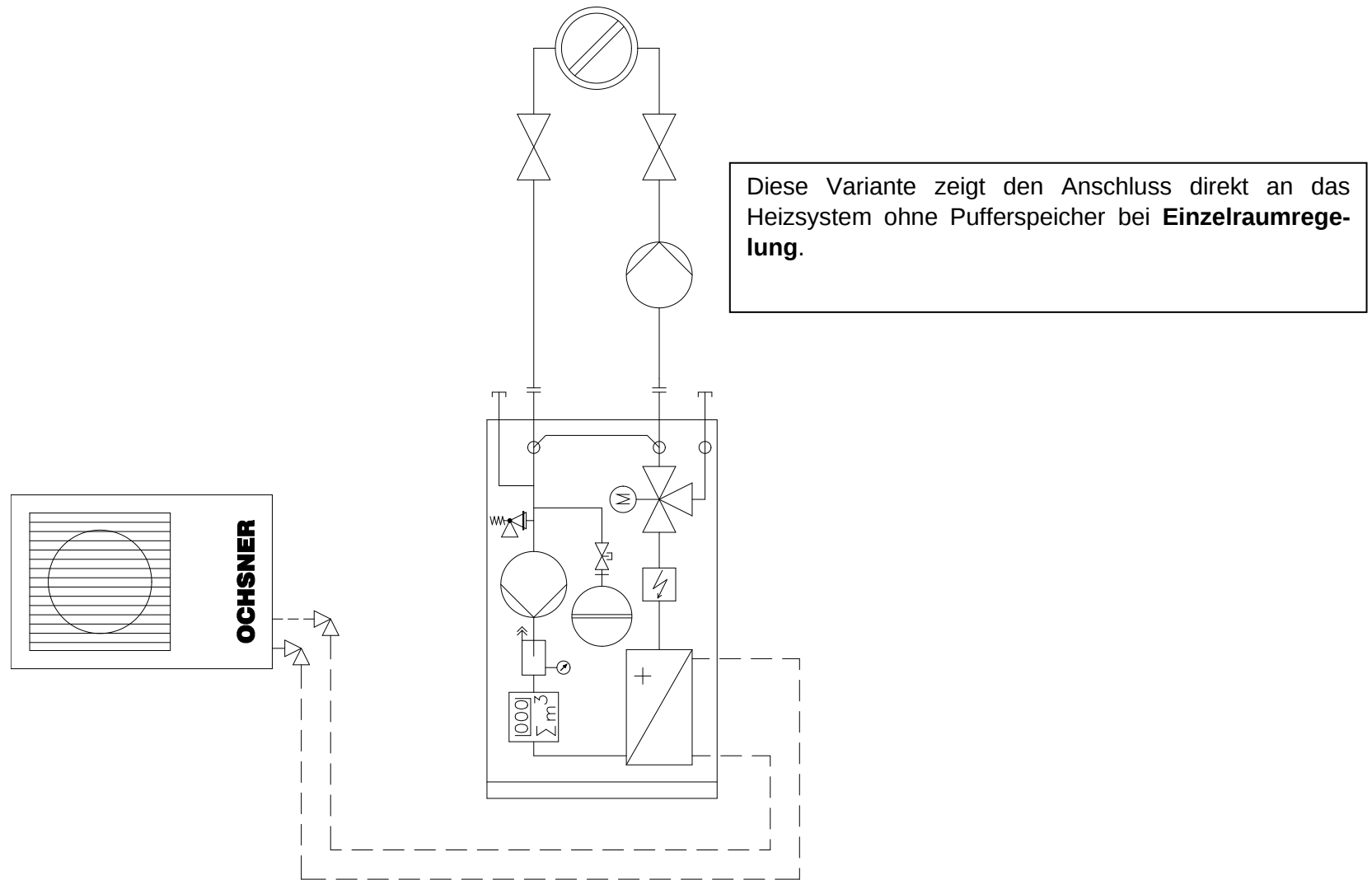
Abbildung 25: Anlagenschema Hydraulik Variante Ia
