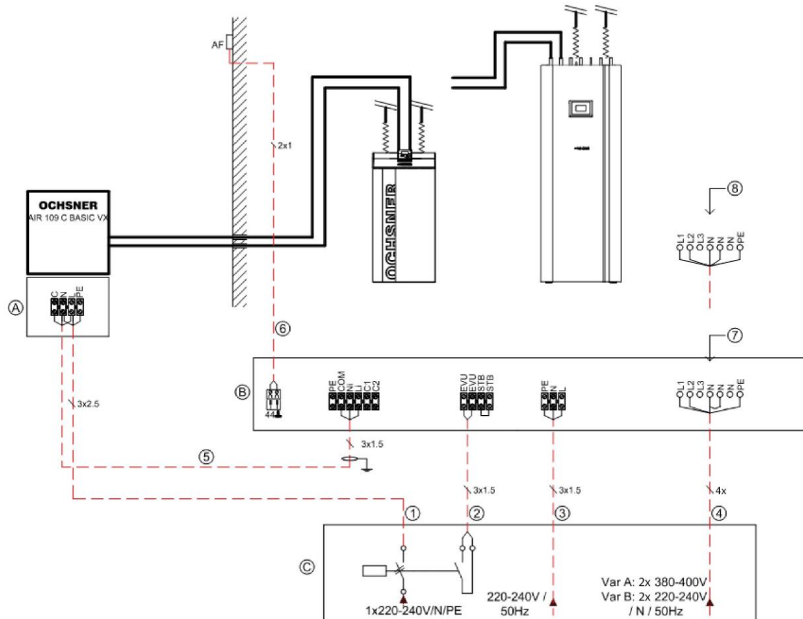
Abbildung 59: Verkabelungsschema AIR BASIC 109
