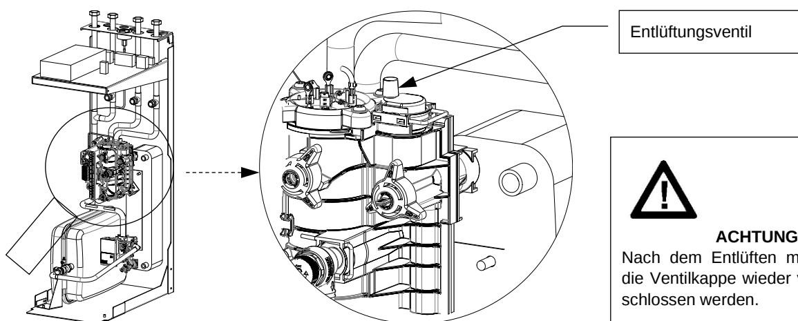
Abbildung 21: Innenteil Entlüftungsventil
