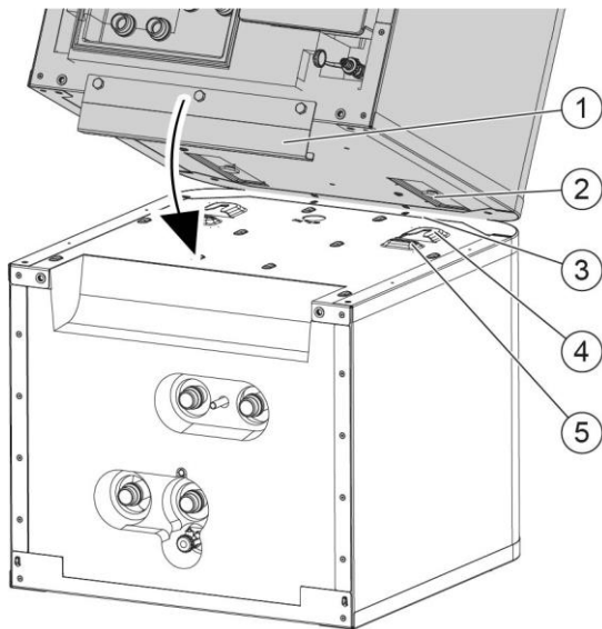
Abbildung 43: Zusammenfügen der Geräteteile 1
