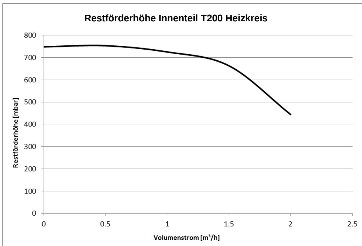
Abbildung 75: Restförderhöhe Innenteil T200 Heizkreis
