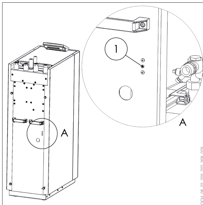
1 Reset-Taster des Sicherheitstemperaturbegrenzers an der Geräterückseite
