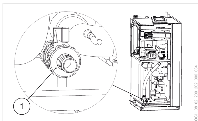
1 Befüllungs- und Entleerungshahn mit Schlauchverschraubung
