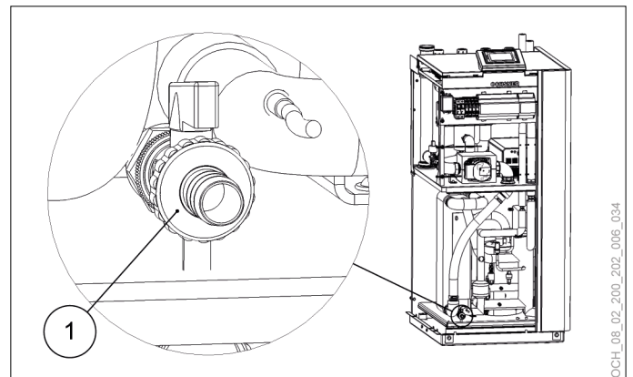
1 Befüllungs- und Entleerungshahn mit Schlauchverschraubung
