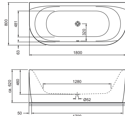
Vorwandwanne Mittelablauf freistehend Frontside bathtub, central drain, free-standing 1800 x 800 x 460 mm
