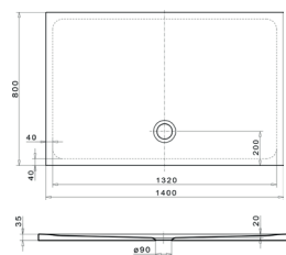
Duschwanne Rechteck shower tray, rectangular 1400 x 800 x 35 mm
