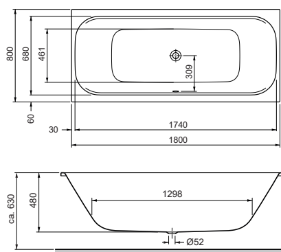
Rechteckwanne Mittelablauf Rectangular bathtub, central drain 1800 x 800 x 480 mm
