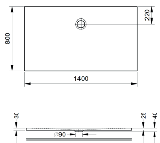
Duschebene Rechteck Shower tray, rectangular 1400 x 800 x 22 mm
