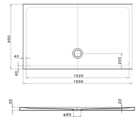
Duschwanne Rechteck shower tray 1600 x 900 x 35 mm
