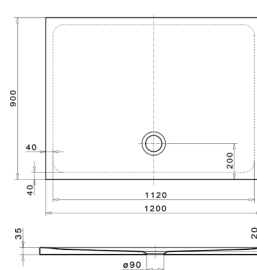
Duschwanne Rechteck shower tray, rectangular 1200 x 900 x 35 mm
