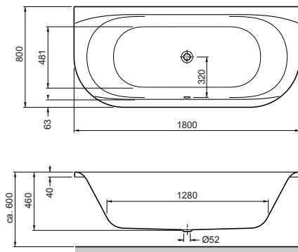
Vorwandwanne Mittelablauf Frontside bathtub, central drain 1800 x 800 x 460 mm
