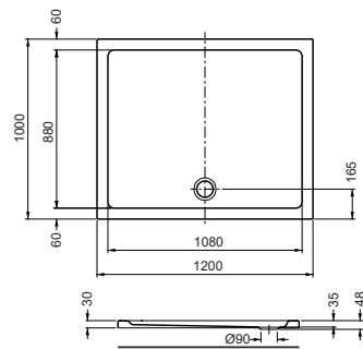
Duschwanne Rechteck Shower tray, rectangular 1200 x 1000 x 35 mm
