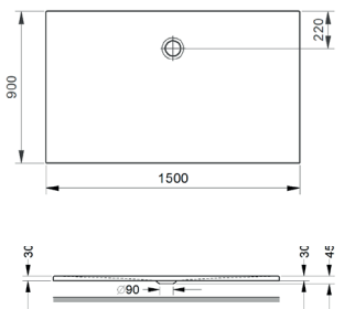
Duschebene Rechteck Shower tray, rectangular 1500 x 900 x 22 mm
