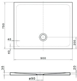
Duschwanne Rechteck shower tray, rectangular 750 x 900 x 35 mm
