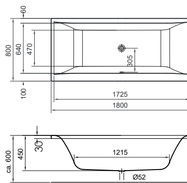
Rechteckwanne Mittelablauf 1800 x 800 x 450 mm Rectangular bathtub, central drain 1800 x 800 x 450 mm
