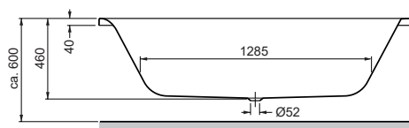
Ecklösung Rechtsausführung 1800 x 800 x 460 mm Corner solution, right-hand model 1800 x 800 x 460 mm
