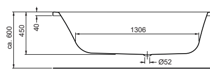
Rechteckwanne mit Duschzone, Überlauf rechts Rectangular bathtub with shower area, overflow on right 1700 x 800 x 450 mm
