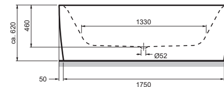
Ecklösung Rechtsausführung mit Untergestell und Schürzenverkleidung Corner solution, right-hand model with underframe and apron panelling 1800 x 800 x 460 mm
