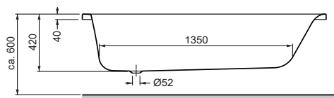
Rechteckwanne mit Duschzone, Überlauf links Rectangular bathtub with shower area, overflow left 1700 x 750 x 420 mm
