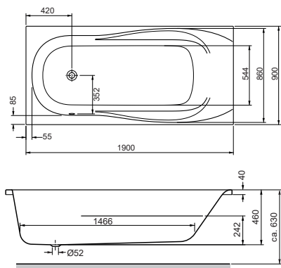
Komfort Körperformwanne Überlauf links Komfort bathtub, overflow left 1900 x 900 x 460 mm
