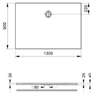
Duschebene Rechteck Shower tray, rectangular 1300 x 900 x 18 mm
