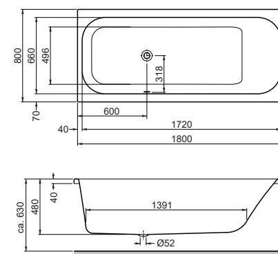
Rechteckwanne mit Duschzone, Überlauf links Rectangular bathtub with shower zone, overflow left 1800 x 800 x 480 mm
