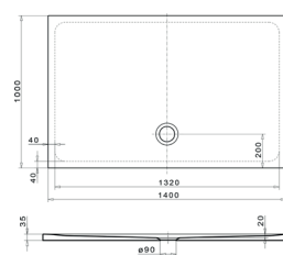
Duschwanne Rechteck shower tray, rectangular 1400 x 1000 x 35 mm
