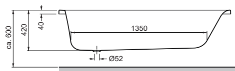
Rechteckwanne mit Duschzone, Überlauf rechts Rectangular bathtub with shower area, overflow right 1700 x 750 x 420 mm
