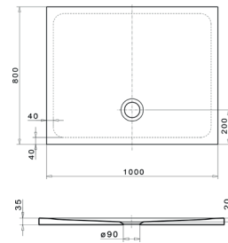
Duschwanne Rechteck shower tray, rectangular 1000 x 800 x 35 mm
