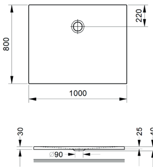
Duschebene Quadrat Shower tray, square 1000 x 800 x 15 mm
