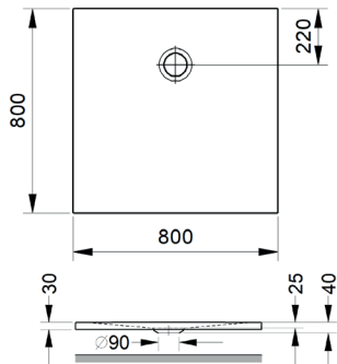
Duschebene Quadrat 800 x 800 x 15 mm Shower tray, square 800 x 800 x 15 mm
