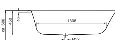
Rechteckwanne mit Duschzone, Überlauf links Rectangular bathtub with shower area, overflow on left 1700 x 800 x 450 mm
