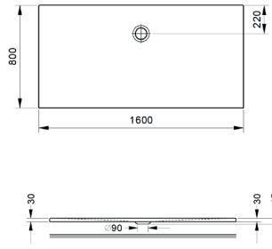
Duschebene Rechteck Shower tray, rectangular 1600 x 800 x 22 mm
