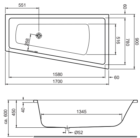
Eckwanne rechts 1700 x 900/600 x 450 mm Corner bathtub, right 1700 x 900/600 x 450 mm
