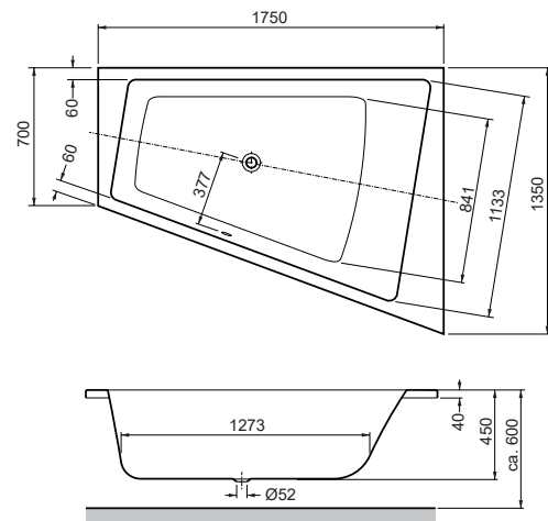
Eckwanne rechts 1750 x 1350/700 x 450 mm Corner bathtub, right 1750 x 1350/700 x 450 mm
