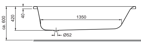
Rechteckwanne mit Duschzone, Überlauf Fußteil Rectangular bathtub with shower area, overflow at foot 1700 x 750 x 420 mm
