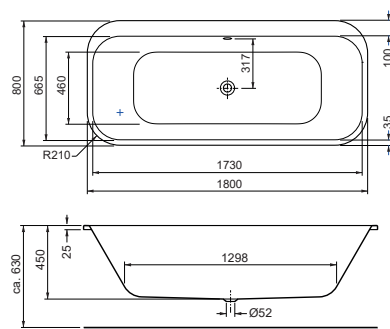
Ovalwanne Mittelablauf 1800 x 800 x 450 mm Oval bathtub, 1800 x 800 x 450 mm
