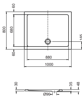
Duschwanne Rechteck Shower tray, rectangular 1000 x 800 x 35 mm
