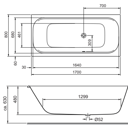
Rechteckwanne mit Duschzone, Überlauf rechts Rectangular bathtub, with shower zone overflow right 1700 x 800 x 480 mm
