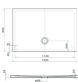
Duschwanne Rechteck shower tray, rectangular 1200 x 800 x 35 mm
