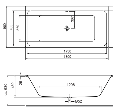
Rechteckwanne Mittelablauf 1800 x 900 x 450 mm Rectangular bathtub, central drain 1800 x 900 x 450 mm
