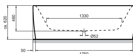
Ovalwanne Mittelablauf freistehend Oval bathtub, central drain, free-standing 1850 x 900 x 460 mm
