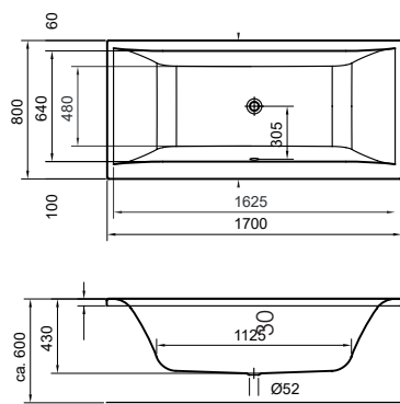
Rechteckwanne Mittelablauf 1700 x 800 x 430 mm Rectangular bathtub, central drain 1700 x 800 x 430 mm
