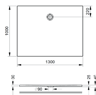
Duschebene Rechteck Shower tray, rectangular 1300 x 1000 x 22 mm
