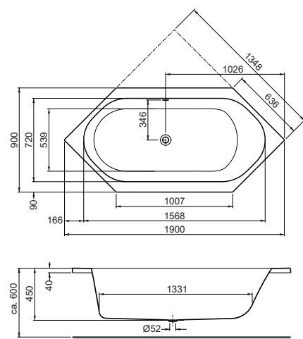
Sechseckwanne, Überlauf rechts Six-sided bathtub, Overflow right 1900 x 900 x 450 mm
