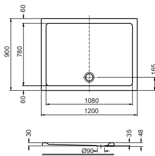
Duschwanne Rechteck Shower tray, rectangular 1200 x 900 x 35 mm
