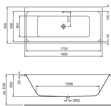
Rechteckwanne Mittelablauf 1800 x 800 x 450 mm Rectangular bathtub, central drain 1800 x 800 x 450 mm
