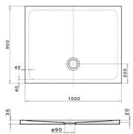
Duschwanne Rechteck shower tray 1000 x 900 x 35 mm
