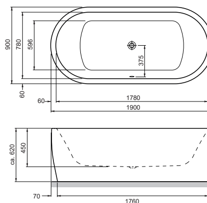
Ovalwanne freistehend 1900 x 900 x 450 mm Oval bathtub, freestanding 1900 x 900 x 450 mm
