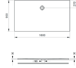
Duschebene Rechteck Shower tray, rectangular 1600 x 900 x 22 mm
