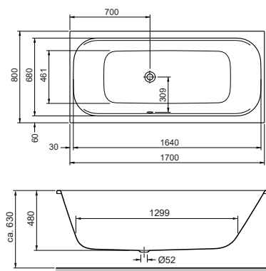
Rechteckwanne mit Duschzone, Überlauf links Rectangular bathtub, with shower zone overflow left 1700 x 800 x 480 mm
