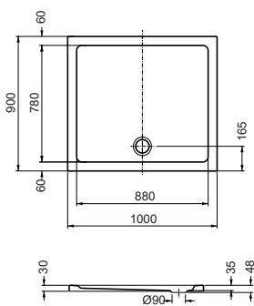
Duschwanne Rechteck Shower tray, rectangular 1000 x 900 x 35 mm
