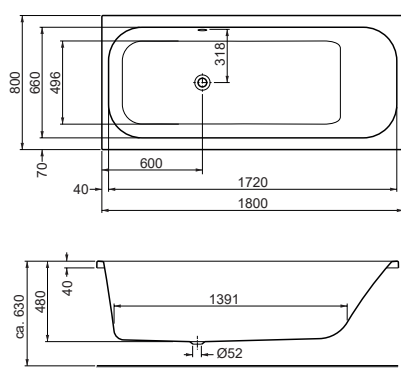
Rechteckwanne mit Duschzone , Überlauf rechts Rectangular bathtub with shower zone, overflow right 1800 x 800 x 480 mm
