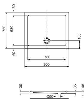
Duschwanne Rechteck Shower tray, rectangular 900 x 750 x 35 mm
