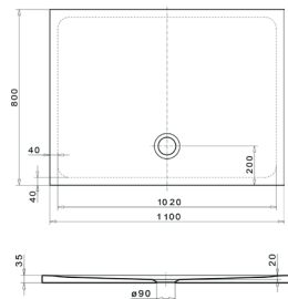
Duschwanne Rechteck shower tray, rectangular 1100 x 800 x 35 mm
