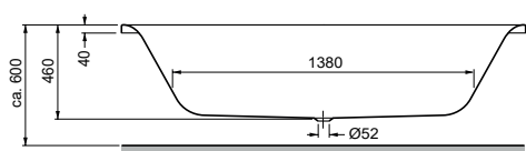
Rechteckwanne Mittelablauf Vasca rettangolare con scarico centrale 1900 x 900 x 460 mm
