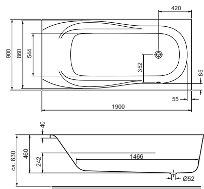
Komfort Körperformwanne Überlauf rechts Komfort bathtub, overflow right 1900 x 900 x 460 mm
