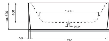
Ecklösung Linksausführung mit Untergestell und Schürzenverkleidung Corner solution, left-hand model with underframe and apron panelling 1800 x 800 x 460 mm
