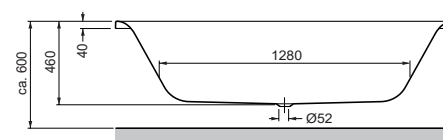
Rechteckwanne Mittelablauf 1800 x 800 x 460 mm Rectangular bathtub, central drain 1800 x 800 x 460 mm
