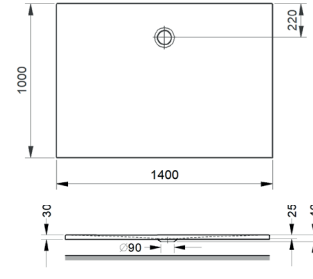
Duschebene Rechteck Shower tray, rectangular 1400 x 1000 x 22 mm
