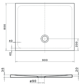
Duschwanne Rechteck shower tray, rectangular 900 x 800 x 35 mm
