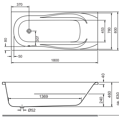
Komfort Körperformwanne Überlauf links Komfort bathtub, overflow left 1800x 800 x 460 mm
