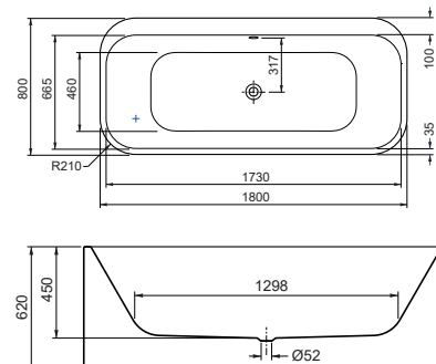
Ovalwanne Mittelablauf 1800 x 800 x 450 mm Oval bathtub, freestanding 1800 x 800 x 450 mm
