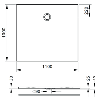
Duschebene Quadrat Shower tray, square 1100 x 1000 x 15 mm
