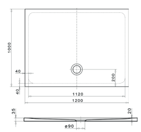
Duschwanne Rechteck shower tray 1200 x 1000 x 35 mm
