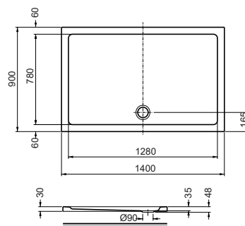
Duschwanne Rechteck Shower tray, rectangular 1400 x 900 x 35 mm
