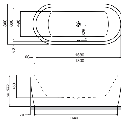
Ovalwanne freistehend mit angeformter Schürze Oval bathtub, freestanding 1800 x 800 x 450 mm
