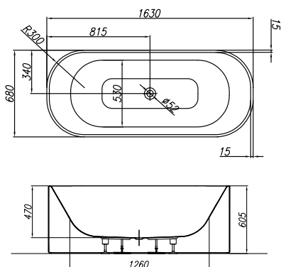
Ovalwanne Mittelablauf freistehend Oval bathtub, central drain free-standing 1630 x 680 x 470 mm
