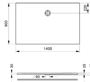
Duschebene Rechteck Shower tray, rectangular 1400 x 900 x 22 mm
