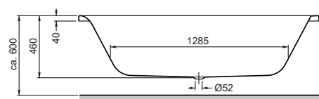
Ecklösung Linksausführung 1800 x 800 x 460 mm Corner solution, left-hand model 1800 x 800 x 460 mm
