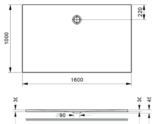
Duschebene Rechteck Shower tray, rectangular 1600 x 1000 x 22 mm
