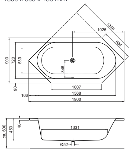
Sechseckwanne, Überlauf links Six-sided bathtub, Overflow left 1900 x 900 x 450 mm
