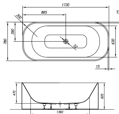
Ovalwanne Mittelablauf freistehend Oval bathtub, central drain, free-standing 1730 x 780 x 470 mm
